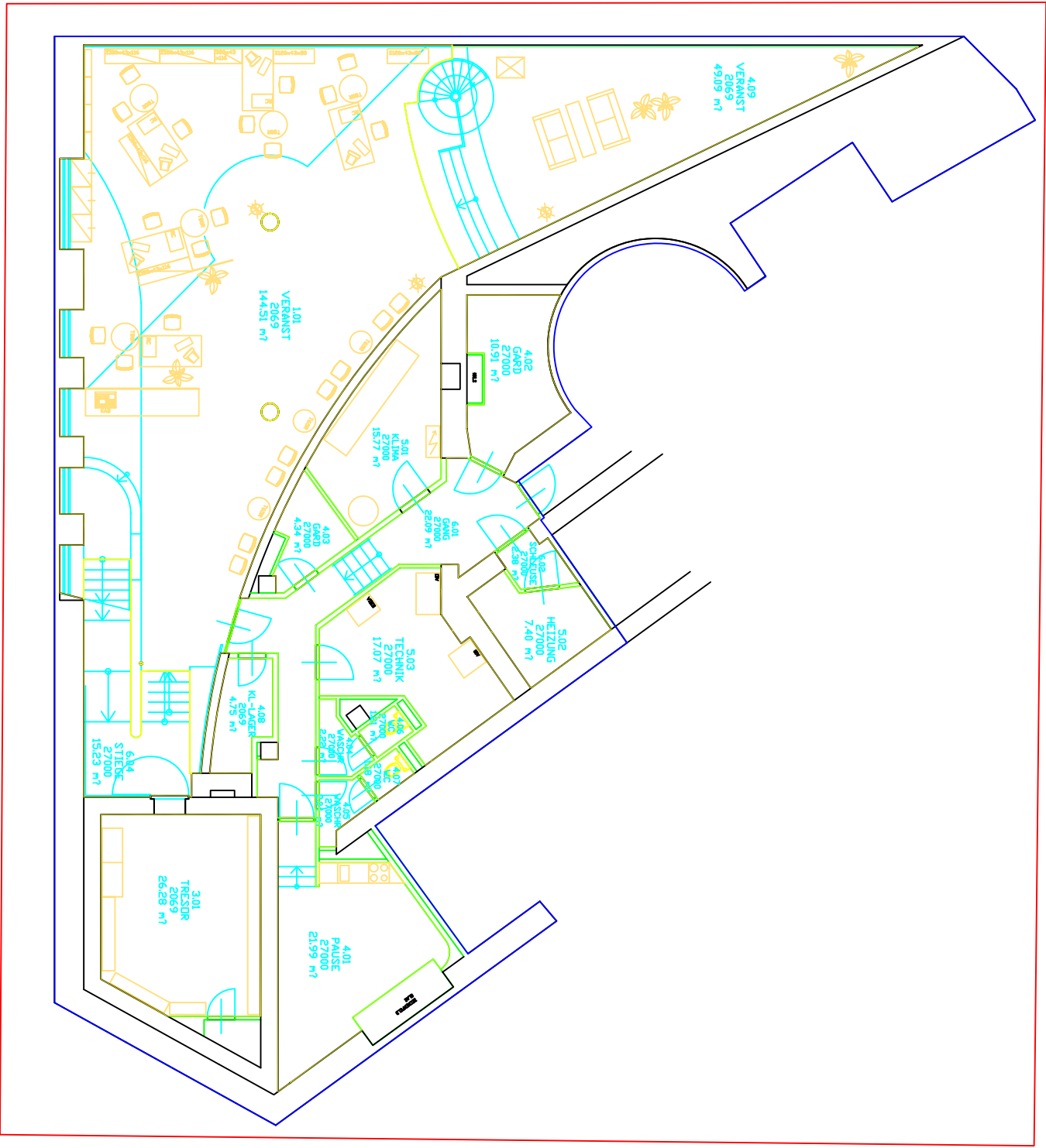
FILIALE GERSTHOF, GRUNDRISS KELLER - IST PLAN
