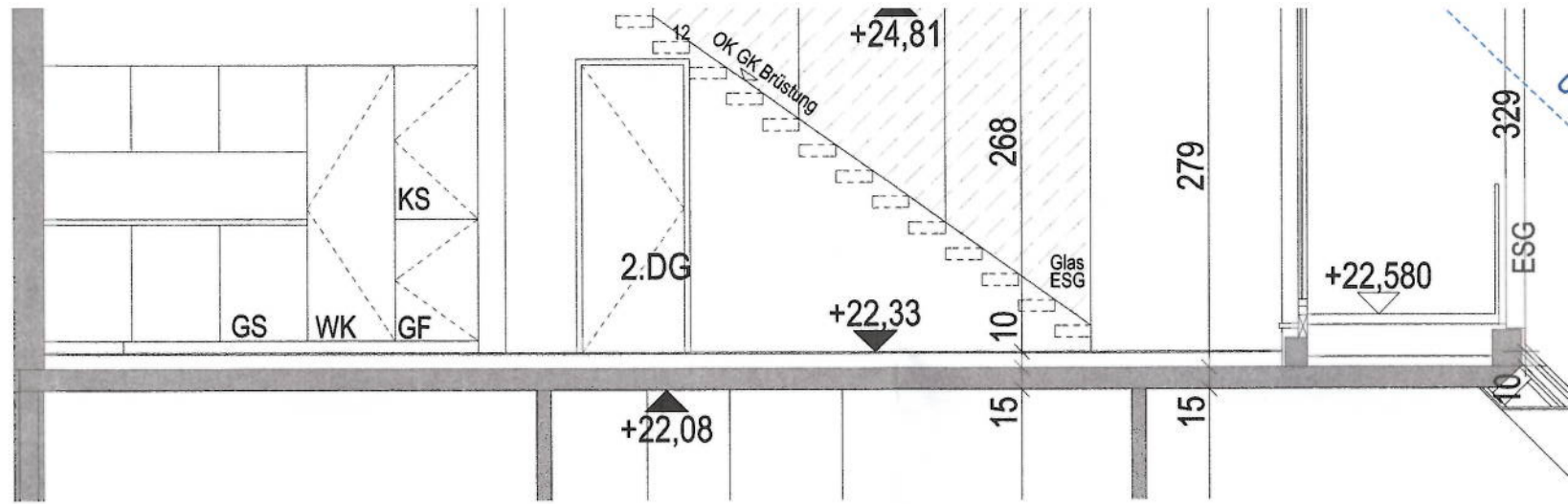
Schnitt C-C
