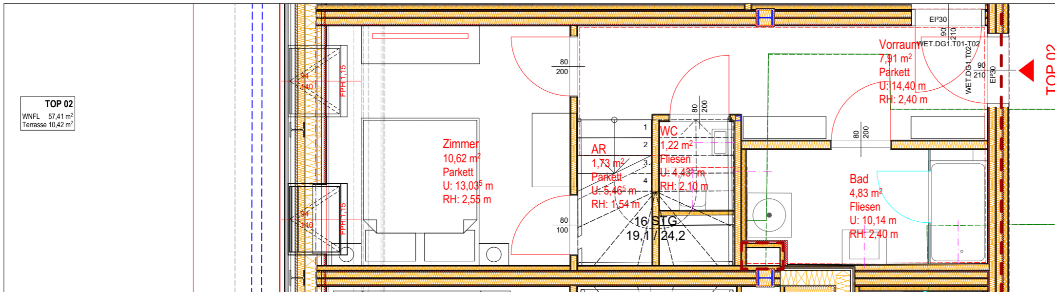
1. DACHGESCHOSS
