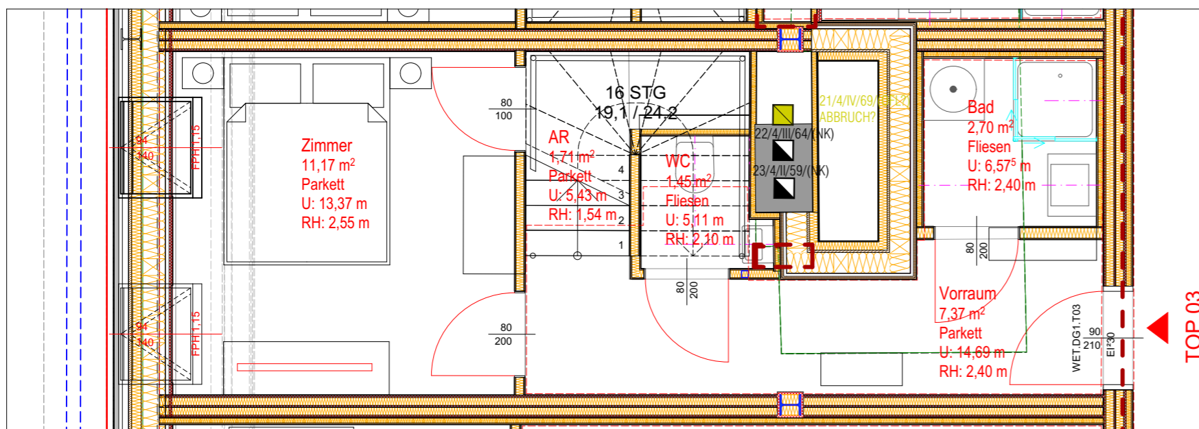
1. DACHGESCHOSS
