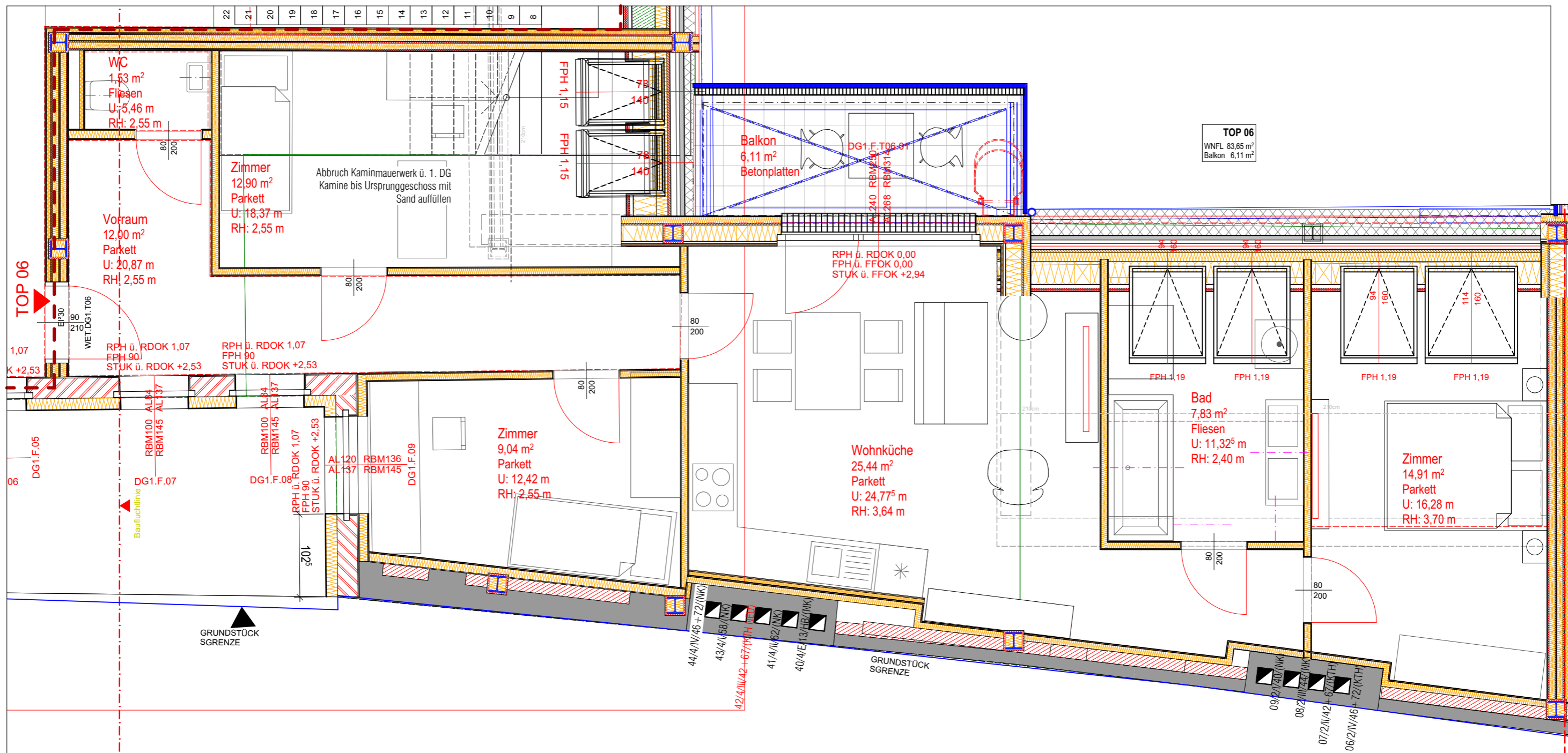
1. DACHGESCHOSS
